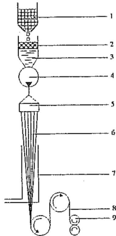
Processo di fabbricazione della fibra multifilamento in PET. 1: grani di PET; 2: riscaldatore; 3: PET fuso; 4: pompa; 5: filiera; 6: filamenti; 7: camera a vapore; 8: fibra multicomponente; 9: bobina di raccolta.
