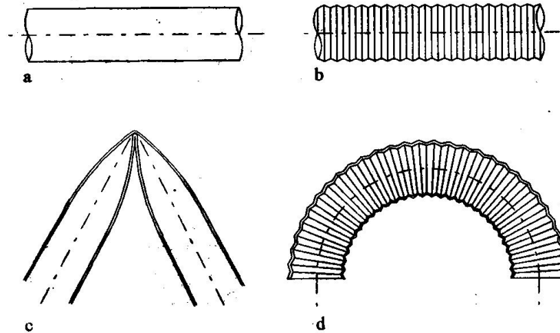
Figura 8.12 Effetto del corrugamento della protesi vascolare sulla sua flessibilità. La protesi non corrugata (a) tende ad occludersi quando viene curvata (c) mentre la protesi corrugata (b) consente curvature senza occlusione del lume (d).
