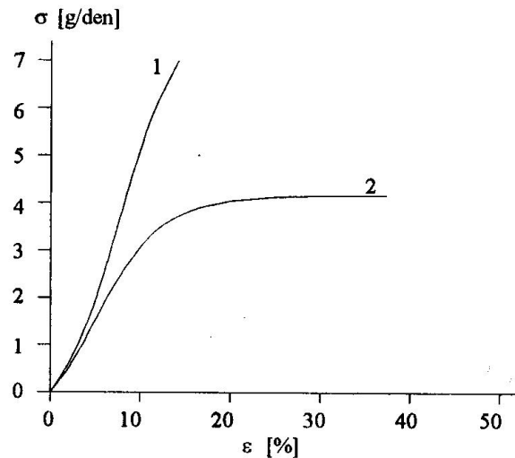
Figura 8.8 Caratteristiche sforzo-deformazione del Dacron stirato (1) e non stirato (2). Lo sforzo è in questo caso espresso in g/den dove den sta per denier che è la misura della sezione di fibra espressa come il peso in grammi corrispondente a 9000 m di lunghezza (da: L Harmon e MS Hoffman 'Fabrication and Testing of Polyester Arterial Grafts' in Vascular Graft Update, ed. KE Kambic, A Kantrowitz e P Sung, ASTM, Philadelphia, 1986).
