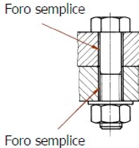
Vite passante
