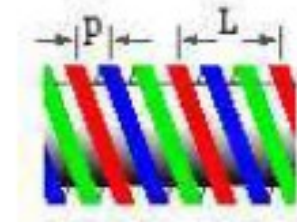
Filettatura a tre principi (avanzamento = 3*passo)
