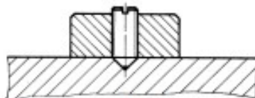
Grano di fermo
