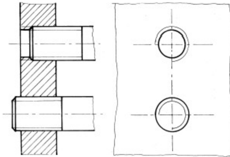
Rappresentazione di accoppiamento vite/madrevite (foro filettato passante)
