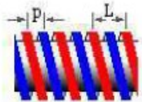
Filettatura a due principi (avanzamento = 2*passo)
